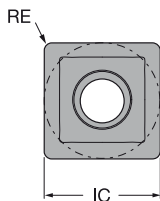
880..P
