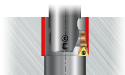
Растачивание
