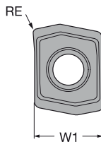
880-01..P
