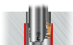
Обратное растачивание
